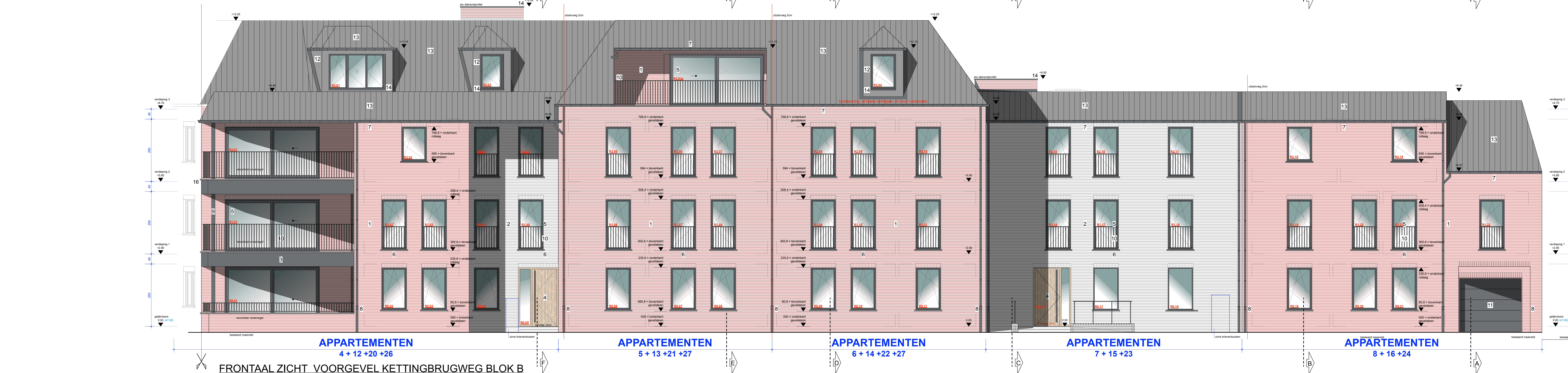
FRONTAAL ZICHT VOORGEVEL KETTINGBRUGWEG BLOK B
